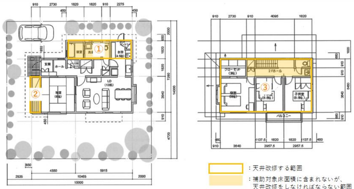
図6-2 天井改修面積算
