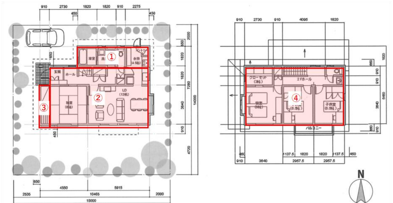
図3 延べ床面積算定
