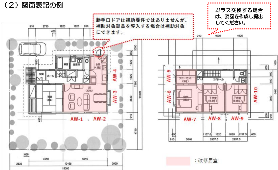
図9 窓改修寸法
